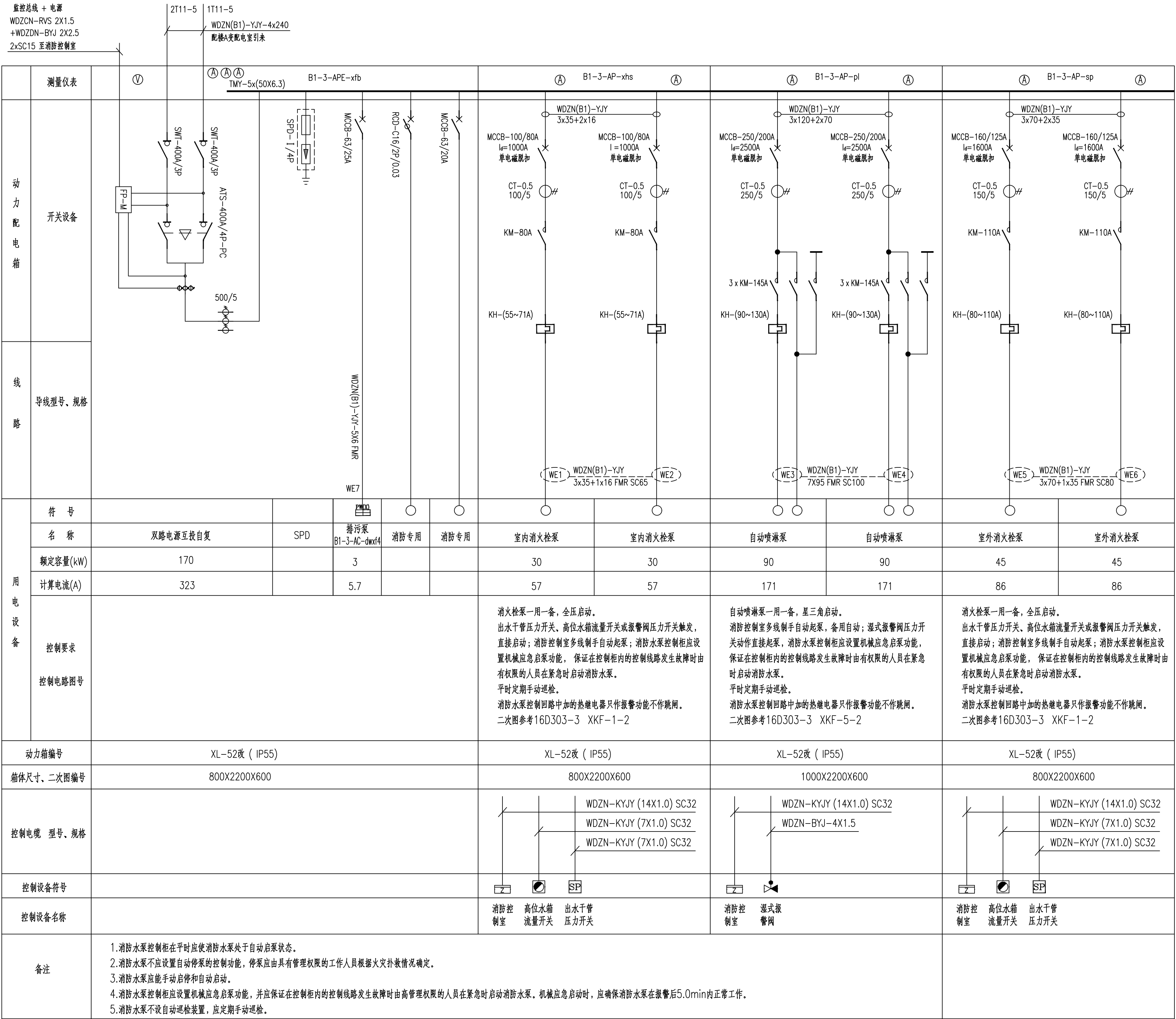
消防水泵房配电系统图
